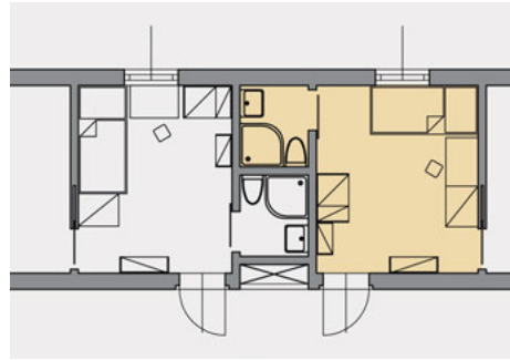
185 Haftraumtypologieentwurf A.S. Variante 2
