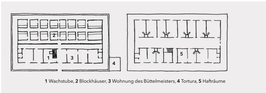
004 J. Furttendach d. Ä., kleines Gefängnis (1634)
