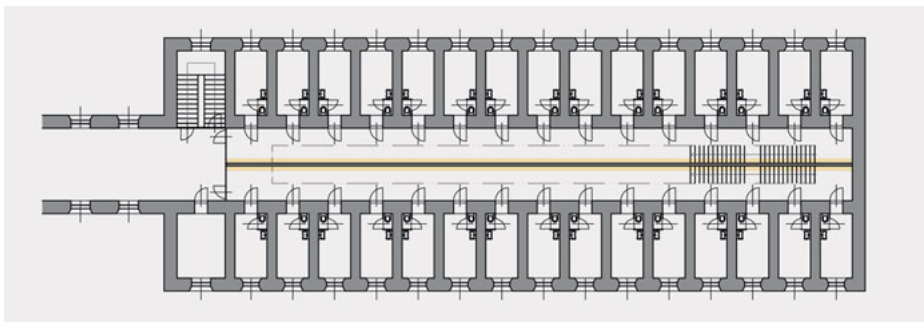
137 Grundriss: Vertikale Teilung
