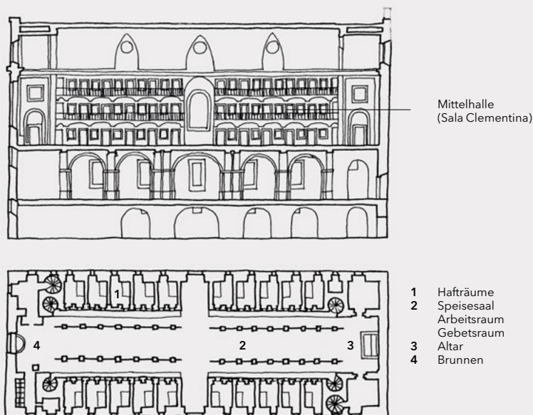
006 Casa di Correzione, Rom (1704)
