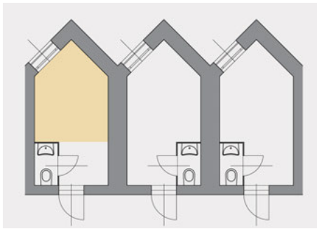
026 Asymmetrischer Wohnraum durch Zackenfassade
