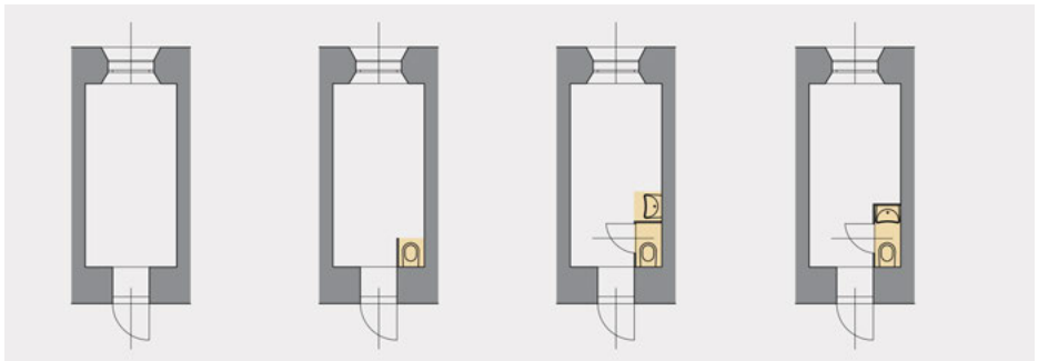
176 Entstehung der Flaschenhalstypologie durch Einbau von Sanitäranlagen
