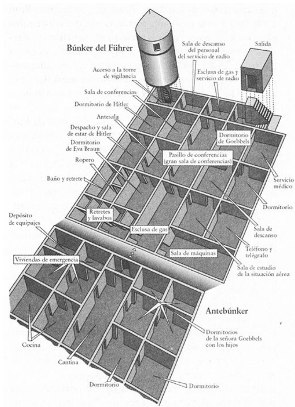
Plano del llamado antebúnker y del búnker del Führer, situado a más profundidad, en el jardín de la cancillería.
