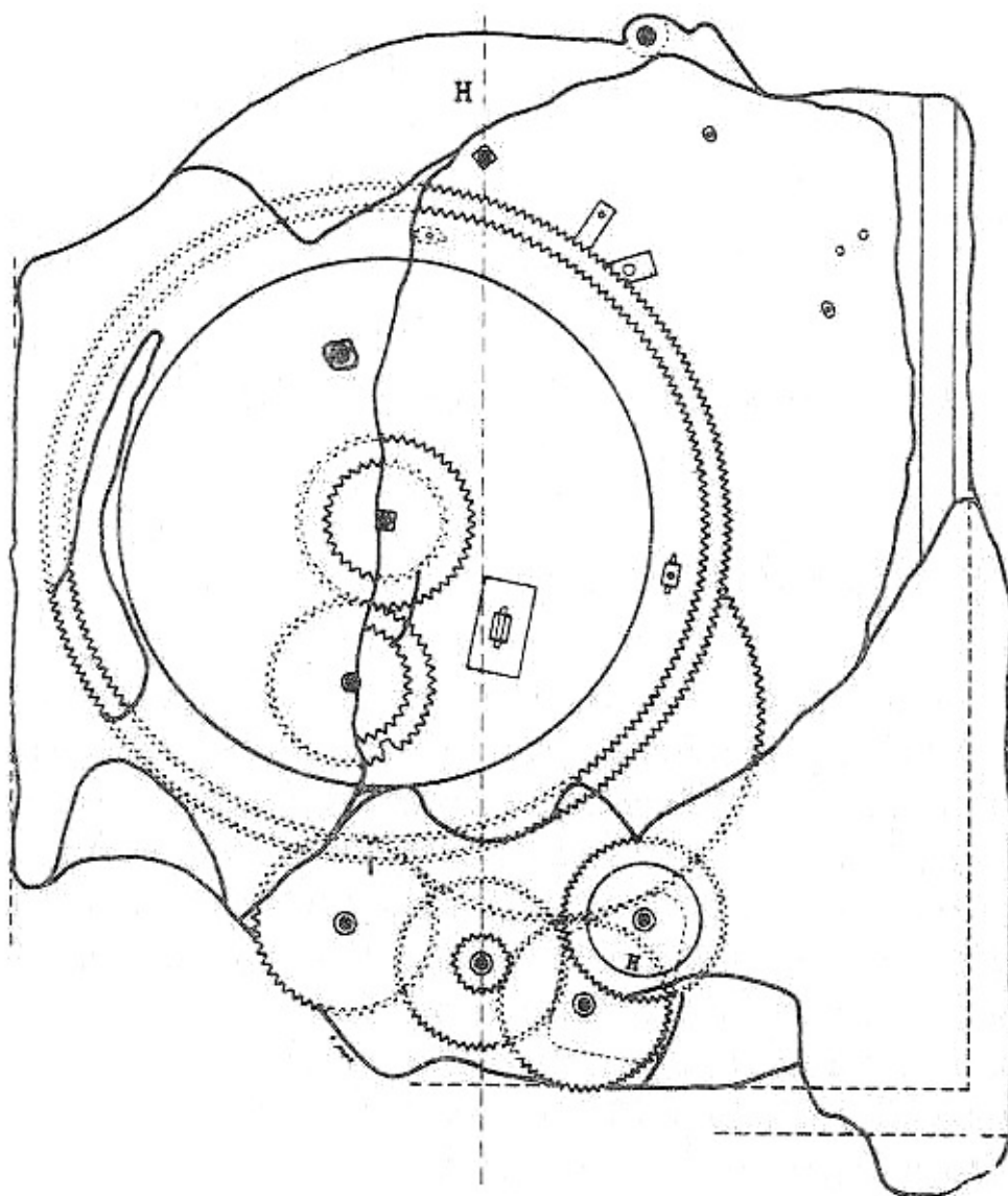
FIGURA 2. Reconstrucción del engranaje mecánico de Antikythera . Esquema del engranaje mecánico de ensamblaje diferencial de Antikythera, reconstruido por D.J. de Solla Price a partir de los cuatro fragmentos de bronce muy corroídos que, según parece, constituyen los restos de 31 ruedas dentadas. A partir de los respectivos números de dientes de los restos, Solla Price sostuvo que la función del instrumento era calendárica, pues le parecía que el mecanismo completo implicaba los números 19 y 235 del ciclo metónico (véase apéndice 2 ). Es posible que este mecanismo formara parte de una colección de «despojos de guerra» transportados por mar a Roma después del saqueo de Atenas por las tropas de Sila en el año 86 a.C.
