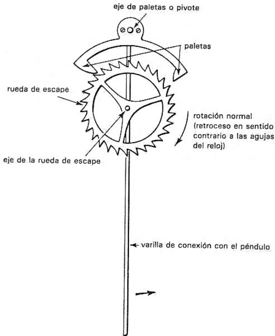
FIGURA 8. El escape de áncora. El escape de áncora consiste en una rueda de dientes afilados y un áncora que lleva, en lugares equidistantes de su eje, dos paletas que van atrapando los dientes de la rueda sucesivamente y cada uno escapa de la acción del otro.
