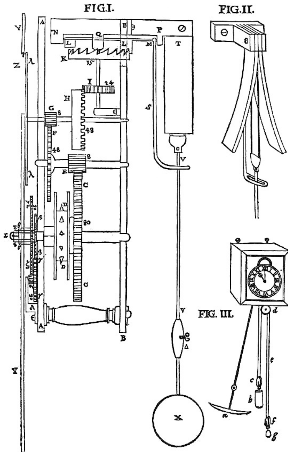
FIGURA 7. El reloj de péndulo de Huygens de 1673. Estos diagramas referentes al reloj de péndulo de Huygens se encuentran en la página 4 de su Horologium Oscilatorium de Motu Pendulorum at Horologia Aptato , publicado en París en 1673 Cum Privilegio Regis y dedicado a Luis XIV. La figura I ilustra los mecanismos del reloj completo con su escape de eje de volante; la figura II las horquillas cicloidales que controlan las oscilaciones del péndulo; y la figura III la apariencia externa del reloj. En este reloj, a diferencia del primer reloj de Huygens, el péndulo colgaba entre horquillas cicloidales, de modo que su tiempo de oscilación era independiente del tamaño del arco de oscilación, propiedad importante para la medida exacta del tiempo.
