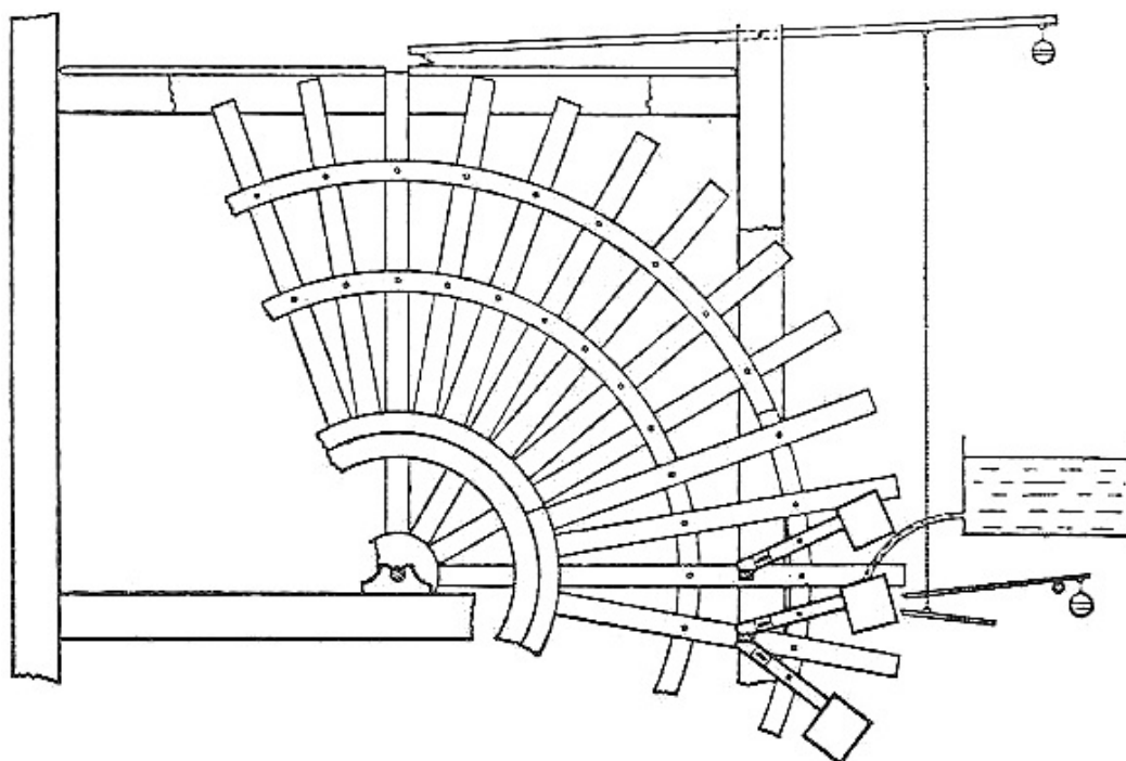
FIGURA I. Reloj de agua medieval chino . Aunque no era un reloj mecánico en el sentido estricto, el reloj de agua de Su Sung incorporaba un modelo muy precoz de escape. Cada 24 segundos el peso del agua que se había derramado a ritmo constante en un cuenco vacío era justo el suficiente para presionar hacia abajo y provocar la rotación de otra espiga de la rueda, situando así otro cuenco vacío bajo la espita. La rueda tenía 36 espas, y daba 100 vueltas en 24 horas.
