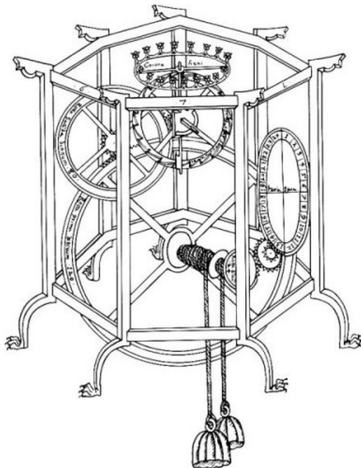
FIGURA 4. Dibujo del reloj astronómico de De'Dondi Fechado en 1461, este dibujo de una parte del reloj astronómico de De'Dondi procede de un manuscrito que se encuentra en la Biblioteca Bodleian de Oxford (MS. Laud Misc. 620, fol. 10v). Este complejo instrumento, terminado en Padua en 1364, estaba accionado por un peso y regulado por un volante de rueda horizontal en forma de corona real. El eje de volante de esta rueda estaba provisto de dos paletas. La superior hacía moverse de uno en uno los 24 dientes de la rueda de escape, que giraba la rueda del eje y del volante, de modo que al mismo tiempo que esta paleta escapaba, la inferior se engranaba. Esta última hacía girar la rueda del eje y del volante en dirección opuesta, y así continuaba el proceso. La rueda del volante tenía un ritmo de 2 segundos. En los últimos años, se han construido varios modelos de este reloj; uno de ellos se encuentra en el Museo de la Smithsonian Institution de Washington, D.C.
