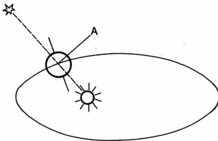
AÑO SIDÉREO
