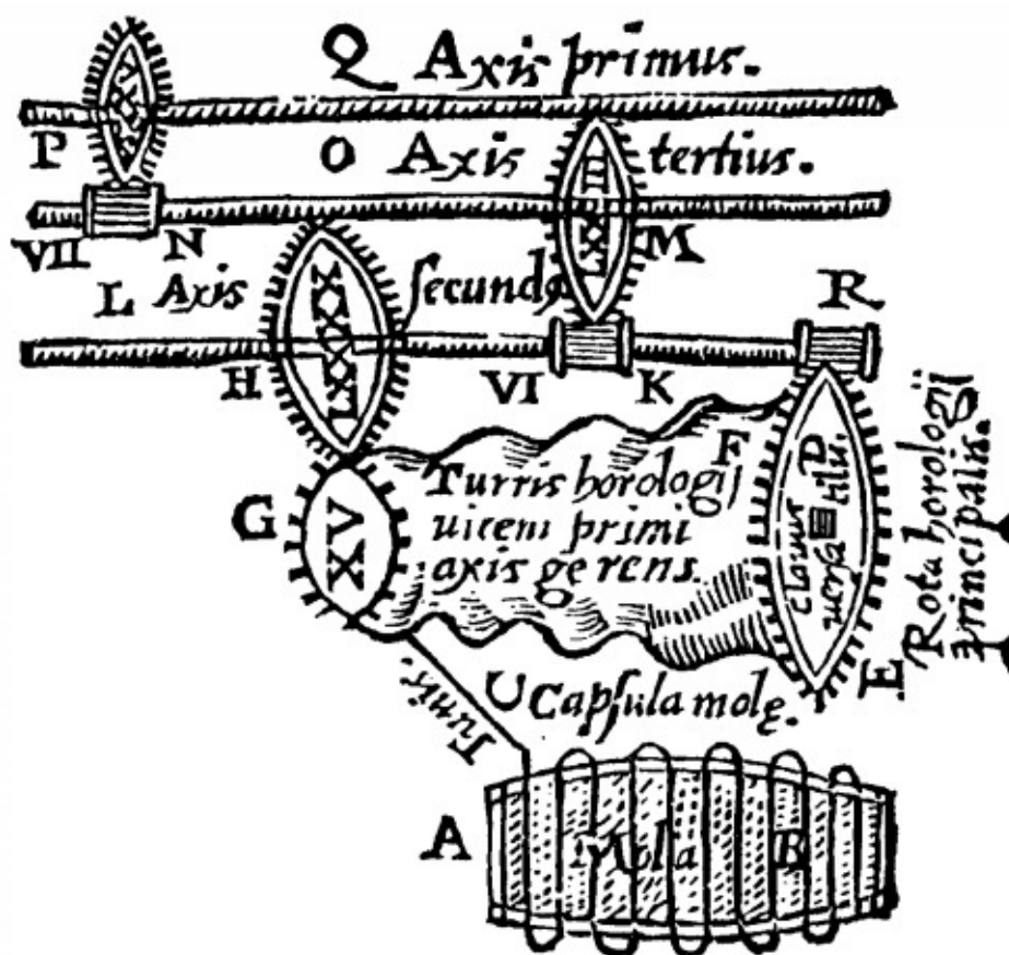
Mecanismo de relojería (De rerum varietate, IX, 47).
