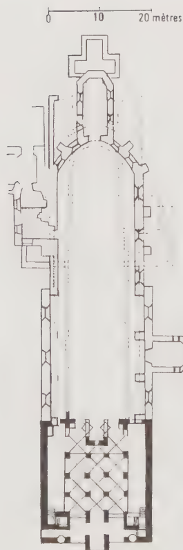
Plan de l'église abbatiale de Corvey
