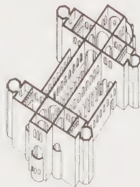
Coupe axonométrique de Saint-Michel de Hildesheim D'après L. Grodecki
