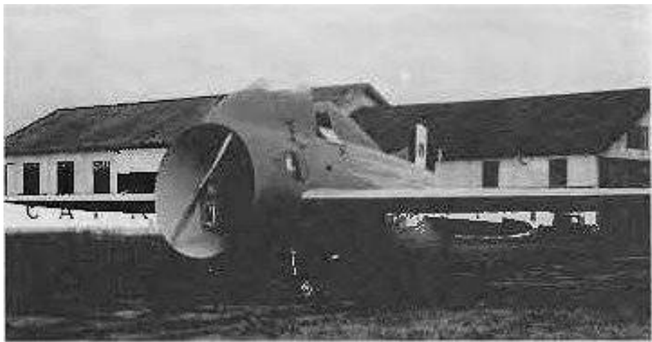
Avion Stipa-Caproni, 1932. Auteur non mentionné. Domaine public.
