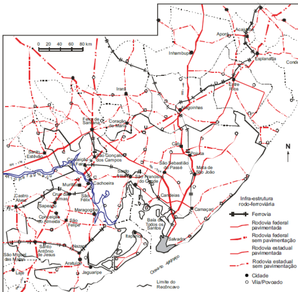
FIGURA 4 - Recôncavo Baiano: estradas e ferrovias - 1960
