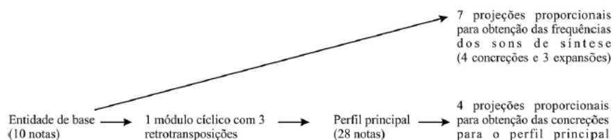
Figura 23 – Representação esquemática da manipulação do espaço harmônico por meio das técnicas dos módulos cíclicos e projeções proporcionais
