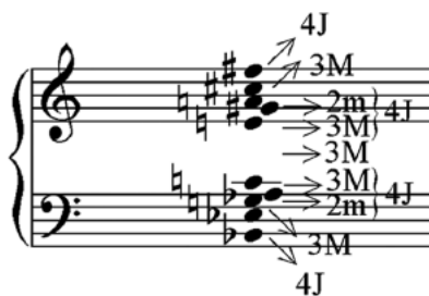
Figura 8 – Simetrias e relações intervalares presentes na entidade harmônica de base utilizada em Parcours de l'Entité (Menezes, 1998)
