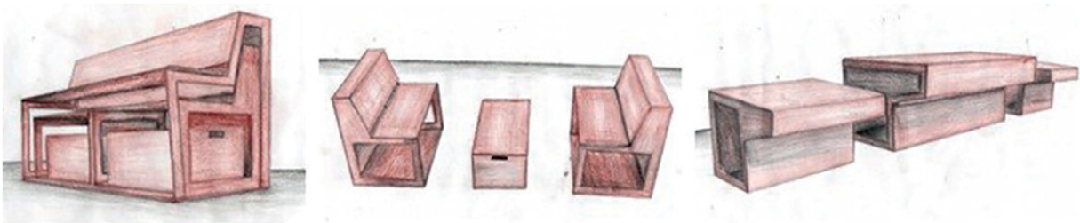
Figura 14 – Croquis do banco modular. Fonte: Ana Paula Z. de Melo (2013).
