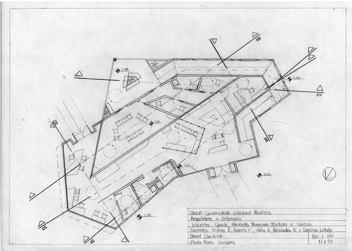
Figura 6 – Planta com layout.
