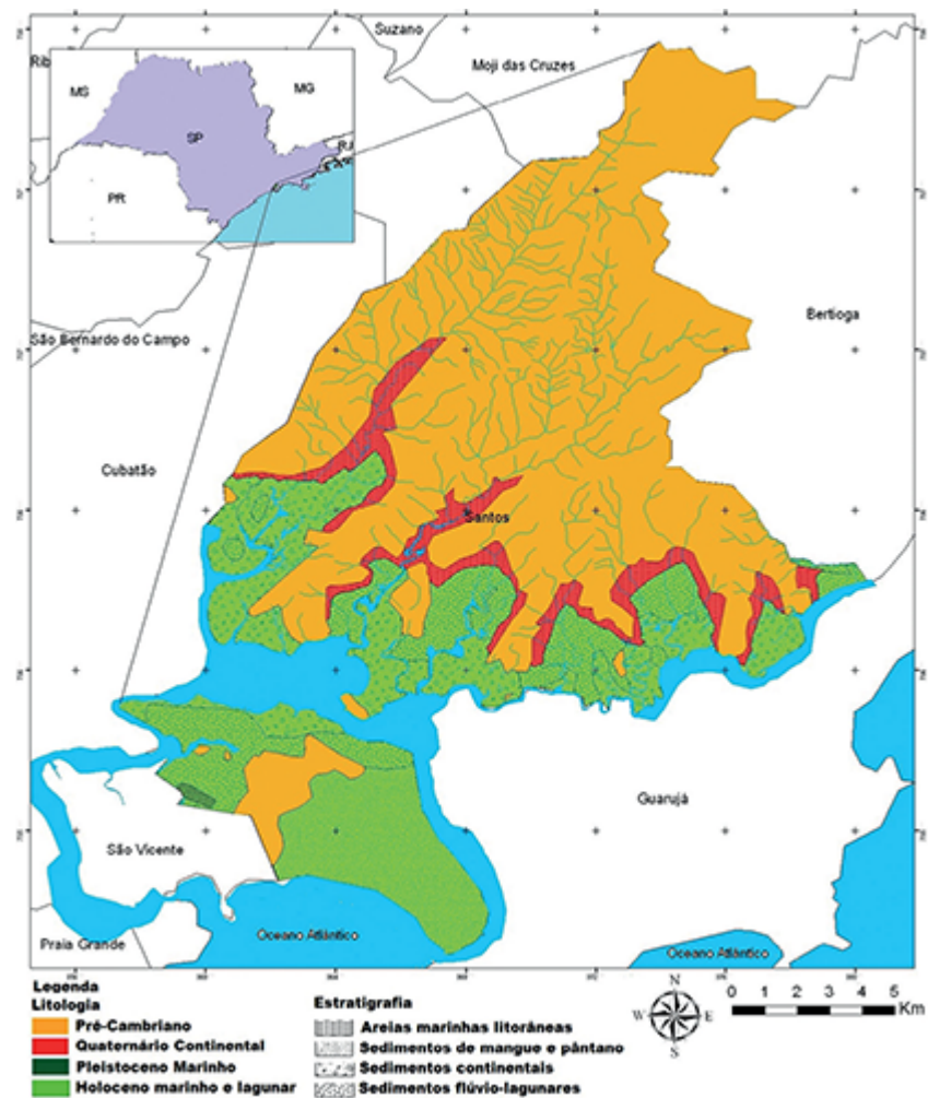
Figura 4.7. Carta Geológica
