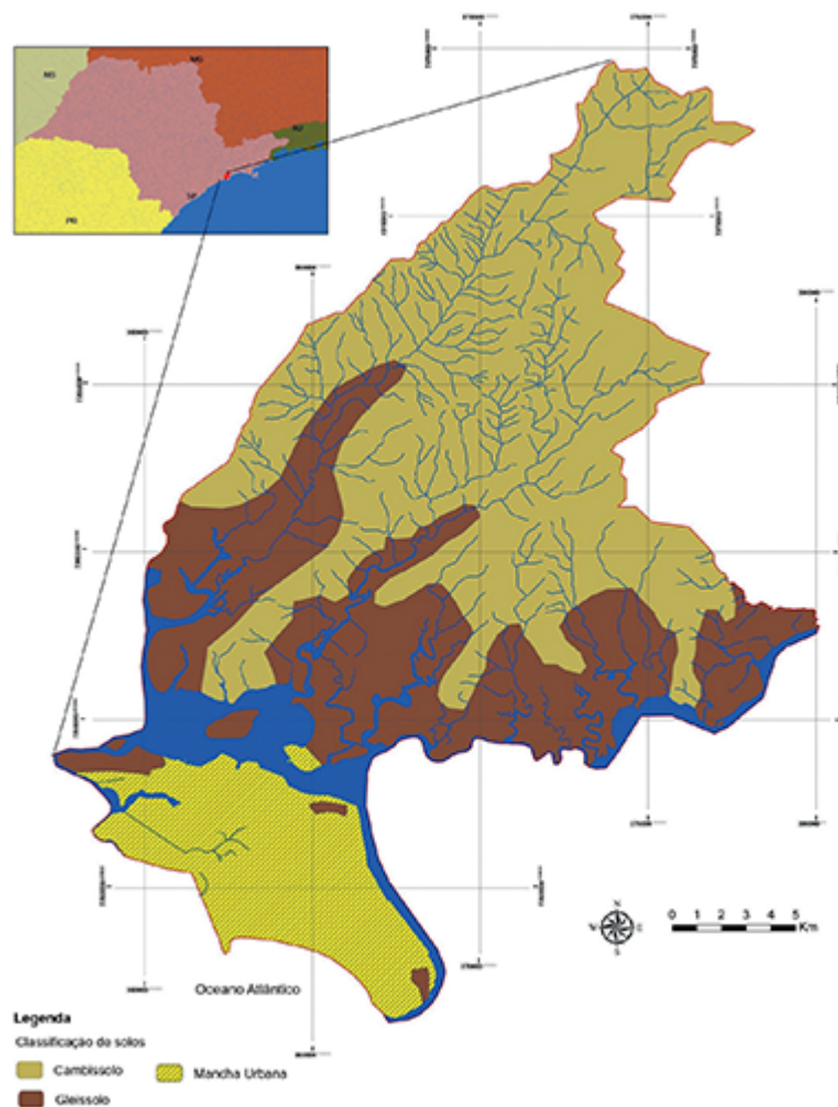
Figura 4.6. Carta Pedológica
