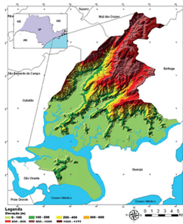
Figura 4.2. Carta Hipsométrica
