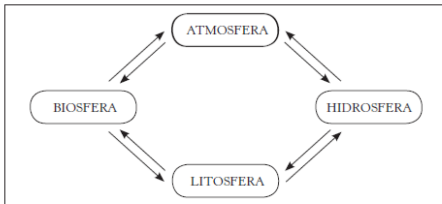
Figura 1: Os subsistemas da Terra. Fonte: Ayoade, 1986 (adaptado de Pitton, S.E.C.)
