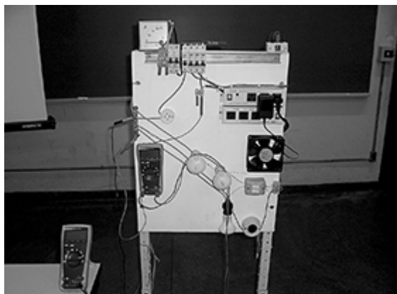
Figura 10 – Circuito elétrico utilizado em experimento demonstrativo.
