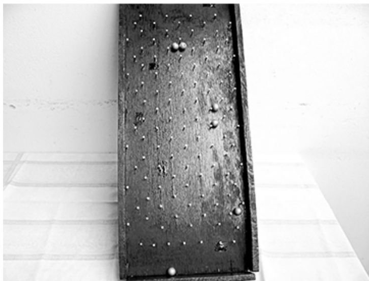
Figura 11 – Maquete tátil-visual-auditiva analógica: corrente elétrica, ddp, resistividade elétrica.
