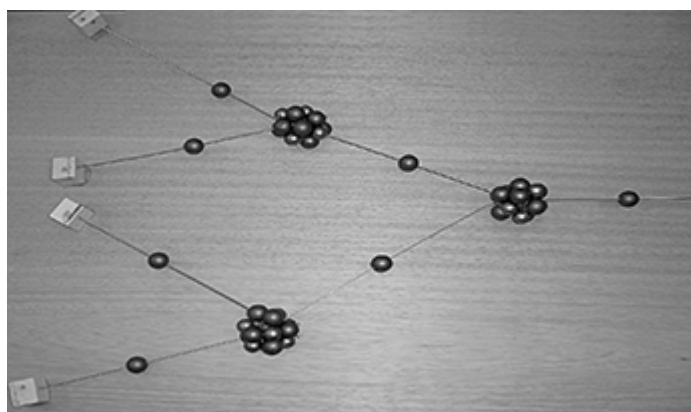
Figura 20 – Registro tátil-visual tridimensional de reação em cadeia (reação nuclear).
