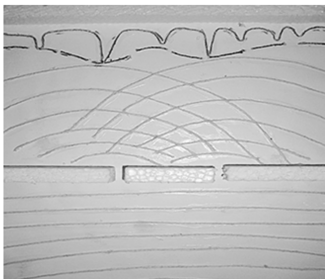
Figura 25 – Registro tátil-visual tridimensional do fenômeno de difração/interferência da luz (difração de Young).
