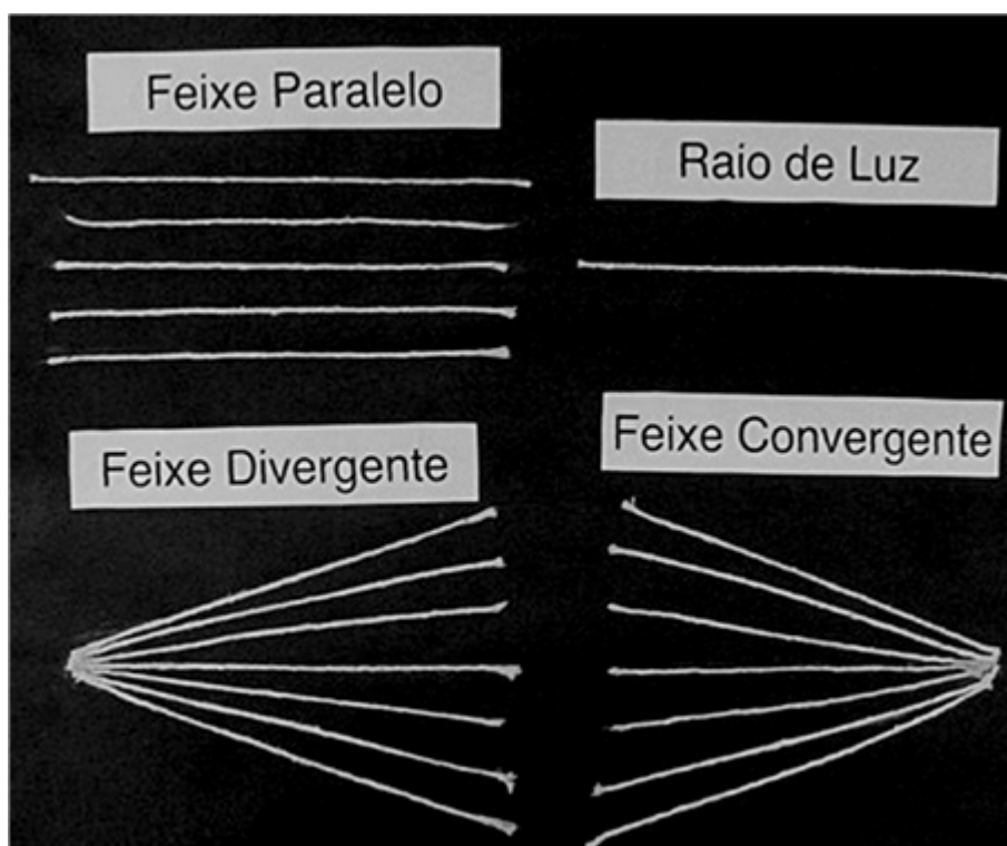
Figura 4 – Registro tátil-visual de raio de luz, raios paralelos, convergentes e divergentes.
