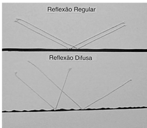
Figura 5 – Representação tátil-visual da reflexão regular e difusa
