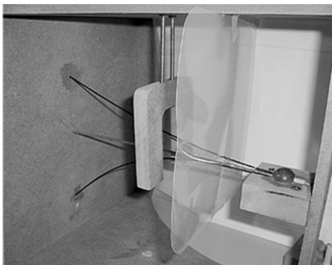
Figura 26 – Registro tátil-visual tridimensional do experimento de Rutherford.
