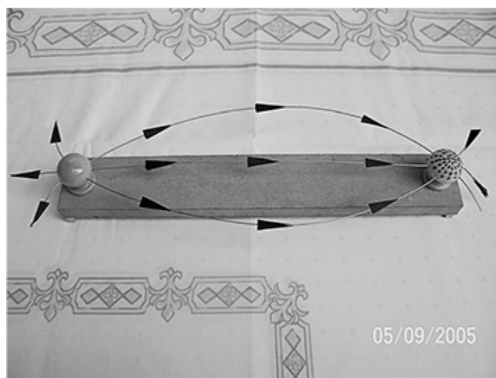
Figura 13 – Maquete tátil-visual de representação de cargas elétricas positiva e negativa e a interação entre suas linhas de força.
