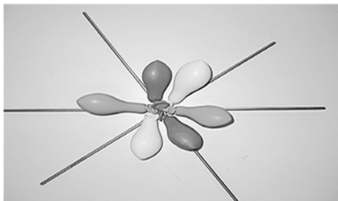
Figura 19 – Registro tátil-visual tridimensional da subcamada P do modelo atômico quântico.
