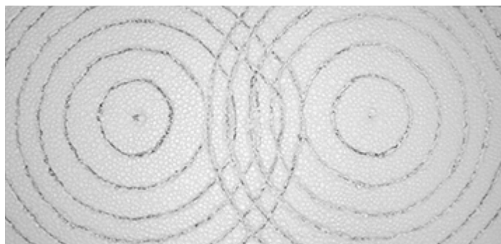
Figura 18 – Registro tátil-visual do fenômeno de interferência de ondas na água.
