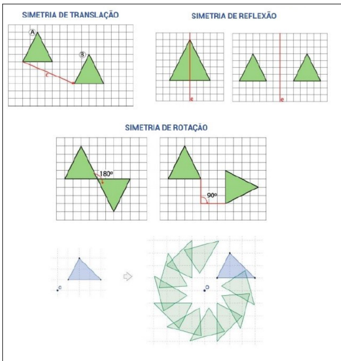
Figura 4 – Isometrias no Plano 7
