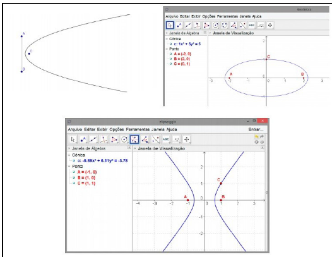
Figura 7 – Parábola, elipse e hipérbole
