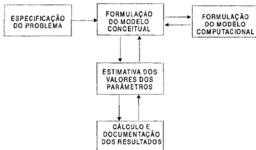
FIGURA 4 - Cinco classes de fatores que afetam a confiabilidade das previsões de modelos matemáticos
