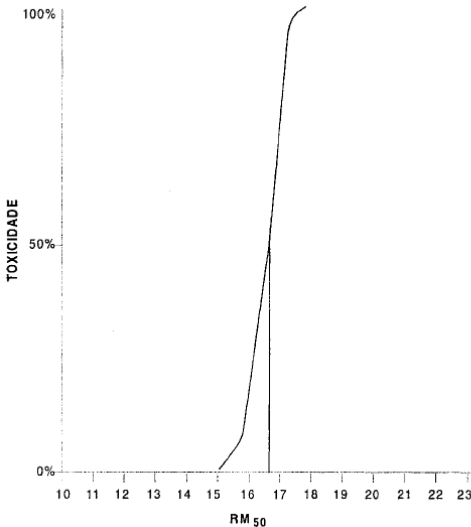
GRÁFICO 2 - Curva teórica dose molecular-resposta mostrando a toxicidade do clorofórmio (em %) versus o número de moléculas do composto (RM 50 )
