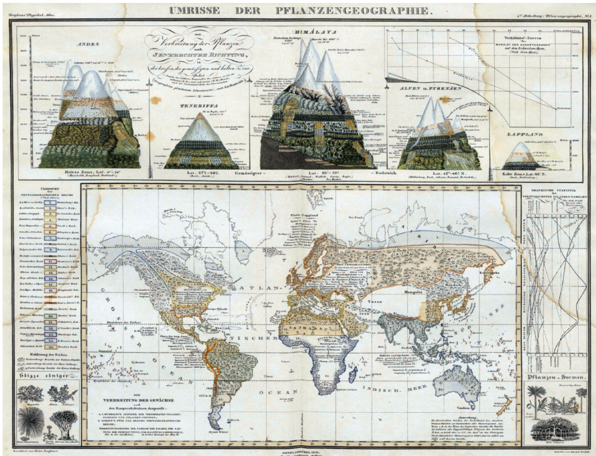
Figura 1 – Forma de representação clássica de Alexander Von Humboldt sobre conexões de fenômenos. Fonte: Physikalischer Atlas (Berghaus, 1845, p.259).
