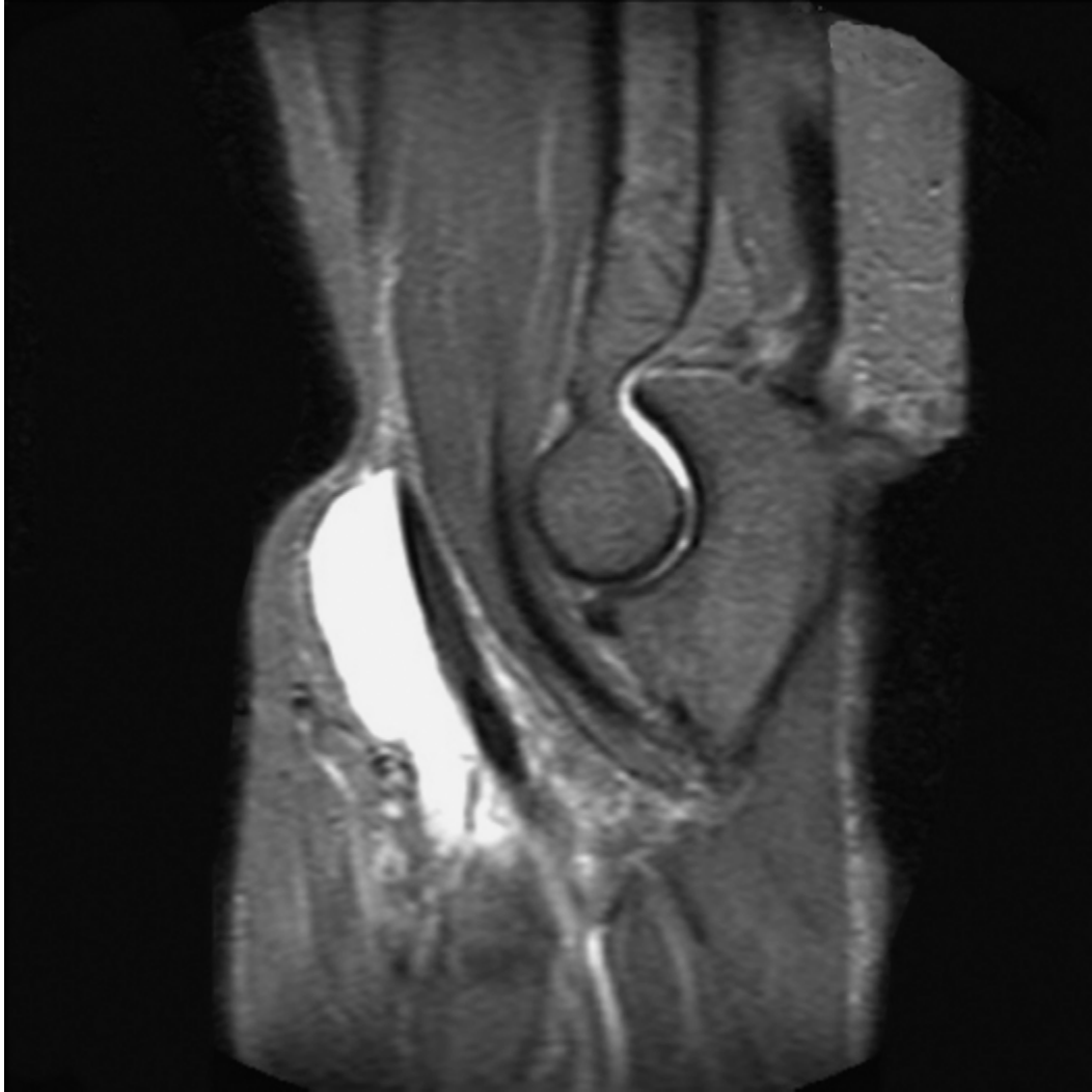
Figura 13.19 STIR sagital.
