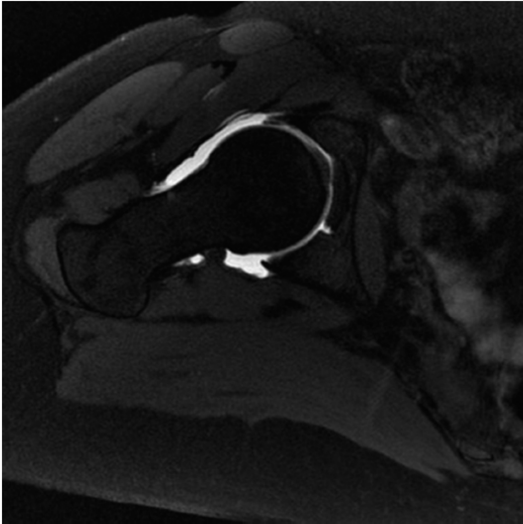
Figura 14.6 Artrografia axial.
