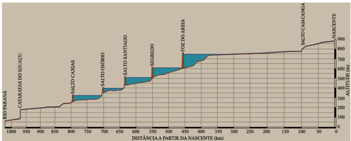
Perfil do rio Iguaçu e seus principais reservatórios , por Jaime Luiz Lopes Pereira (adaptado de Júlio Júnior, Bonecker e Agostinho, 1997).
