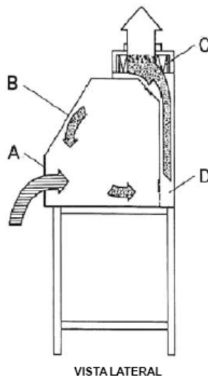
FIGURA 4.1 — Cabine de Segurança Biológica classe I: (A) abertura frontal; (B) vidraça corrediça; (C) filtro HEPA para exaustão; (D) espaço de exaustão Fonte: Brasil (2001), com modificações.
