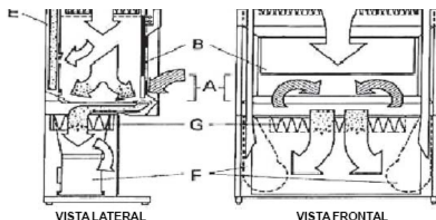
FIGURA 4.2b — Cabine de Segurança Biológica classe II tipo B1 (desenho clássico): (A) abertura frontal; (B) vidraça corrediça; (C) filtro HEPA para exaustão; (D) filtro HEPA para o suprimento de ar; (E) espaço de exaustão com pressão negativa; (F) ventilador; (G) filtro HEPA adicional para o suprimento de ar Obs.: exaustor da cabine necessita ser conectado ao sistema de exaustores do edifício. Fonte: Brasil (2001), com modificações.
