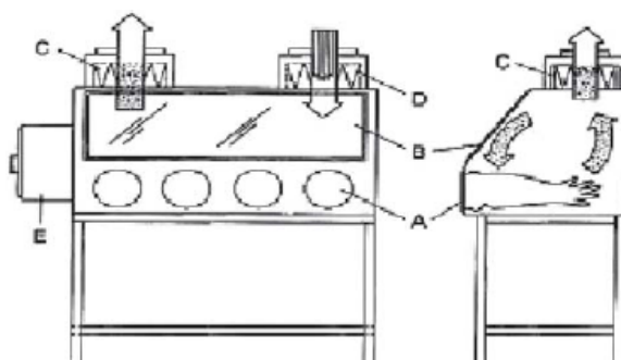
FIGURA 4.3 — Cabine de Segurança Biológica classe III: (A) compartimento para fixação de luvas longas de borracha à cabine; (B) vidraça corrediça; (C) filtro HEPA para exaustão; (D) filtro HEPA para o suprimento de ar; (E) autoclave dupla saída na extremidade ou caixa de passagem da cabine.
