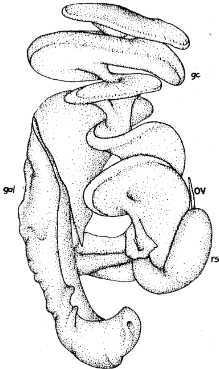
Figura 17: Glândula de P. Lineata : gal : glândula de albume; gc : glândula da casca em espiral; ov : oviduto; rs : receptáculo seminal.
