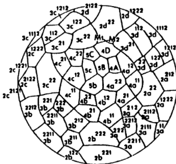
FIGURA 2-17: Estádio de 106 blastômeros (pólo vegetativo), 19 horas após a primeira clivagem. O mesoblasto primário M1, e M2 com pequena superfície externa
