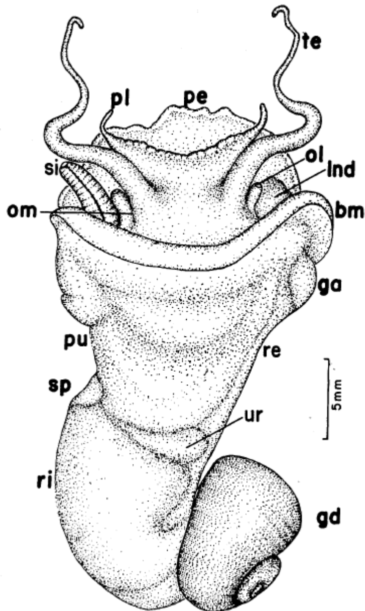
Figura 6: P. lineata , animal retirado da concha. bm: borda do manto; ga: glândula anal; gd: glândula digestiva; lnd: lóbulo nugal direito; ol: olho; om: omatóforo; pe: pé; pl: palpo labial; pu: pulmão; re: reto; ri: rim; sp: saco espermático; si: sifão; te: tentáculo; ur: ureter
