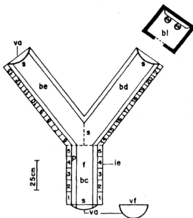
FIGURA 4: Representação esquemática de um aquário em forma de Y usado para estudar a orientação de B. glabrata em relação a luz. bc. = braço central; bd. = braço direito; be. = braço esquerdo; bl. = caixa com luz; f. = fundo; ie. = identificação externa das áreas; p. = paredes; s. = sítio de medição de temperatura; va. = vasilhame de acrílico; vf. = vista frontal
