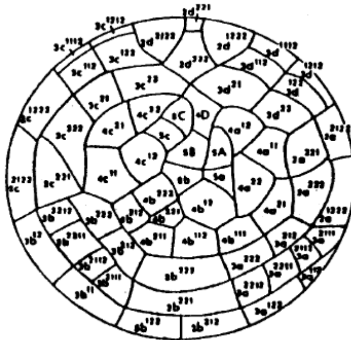
FIGURA 2-19: Estádio de 130 blastômeros (pólo animal), 21:30 horas após a primeira clivagem
