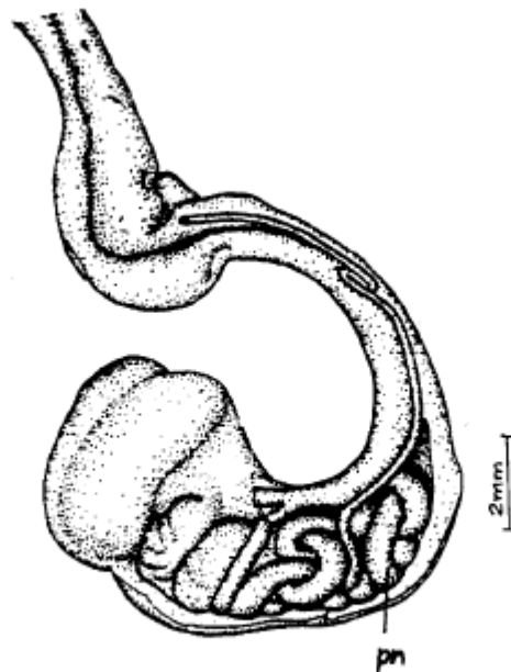
Figura 11. P. Lineata . Pênis enovelado dentro da bolsa: pn : pênis.
