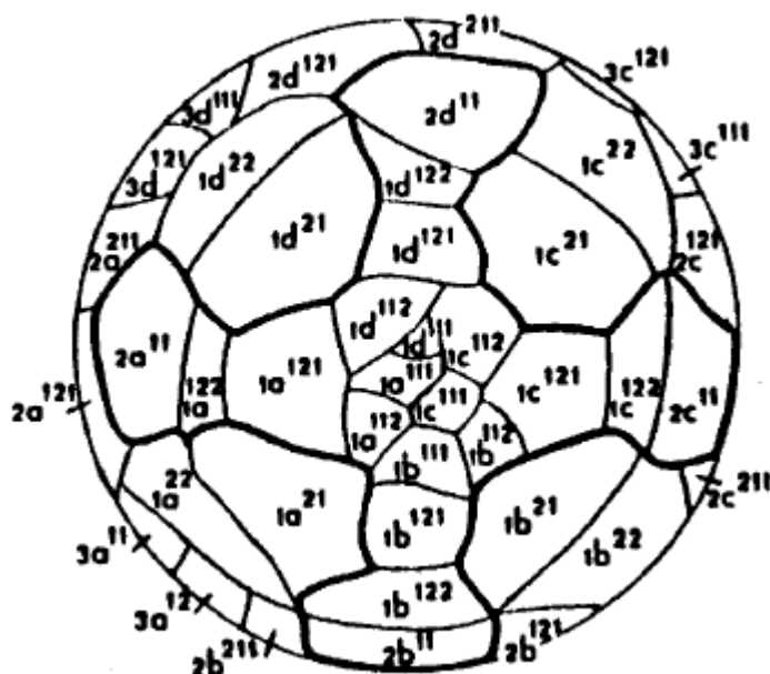
FIGURA 2-17: Estádio de 106 blastômeros (pólo vegetativo), 19 horas após a primeira clivagem. O mesoblasto primário M1, e M2 com pequena superfície externa
