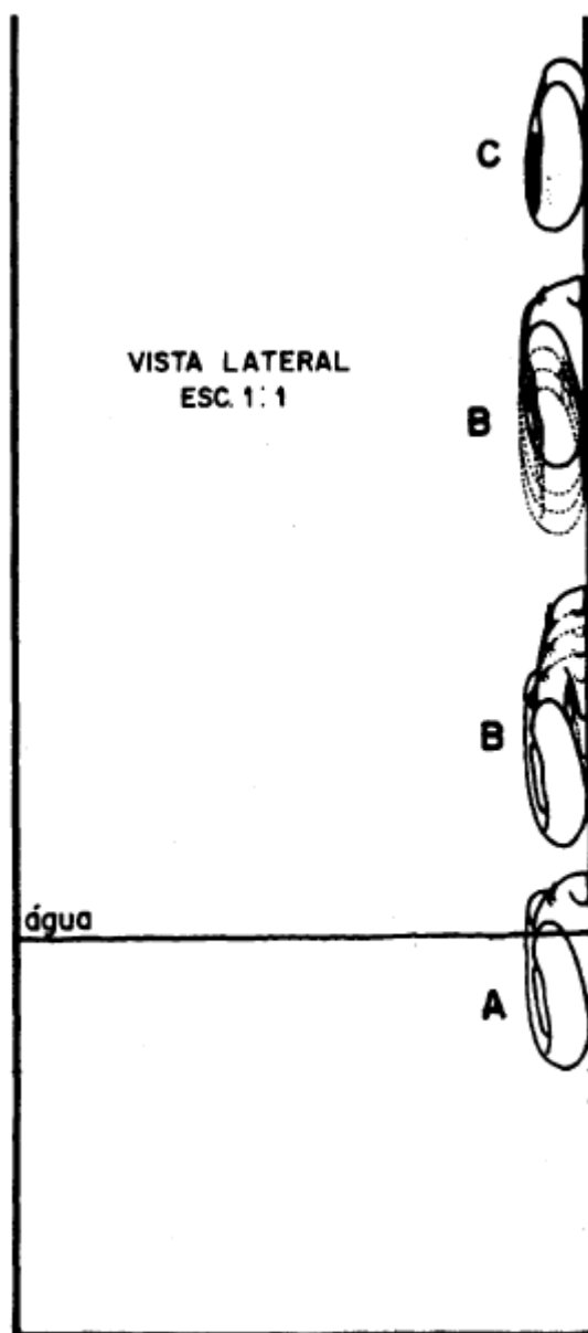
FIGURA 29: Seqüência de movimentos, deslocamentos e posturas que caracterizam a saída da água. (A) Estando o caramujo na superfície, ele rompe a película da água. A concha passa a ter uma postura pendente; (B) O caramujo prossegue no seu deslocamento se arrastando, com a concha pendente e a massa cefalopodal aderida a parede lateral do aquário; (C) Uma vez atingida uma certa altura acima do nível da água, o caramujo aí permanece aderido ao vidro lateral do aquário, pela face esquerda da concha
