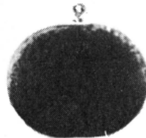
FIGURA 1-6/7: Os dois blastômeros continuando com a superfície de contato, 26 e 38 minutos respectivamente
