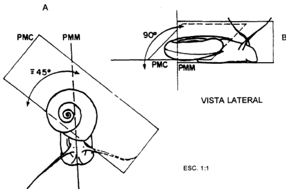
FIGURA 12: Concha pendente. (A) rotação da concha para a esquerda do observador (ângulo podendo variar entre 45^\circ e 90^\circ ); (B) inclinação da concha para a direita do observador (ângulo de 90^\circ ). PMC - plano mediano da concha; PMM - plano mediano da massa cefalopodal
