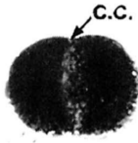
FIGURA 1-10: Segunda clivagem, 80 minutos após a primeira clivagem
