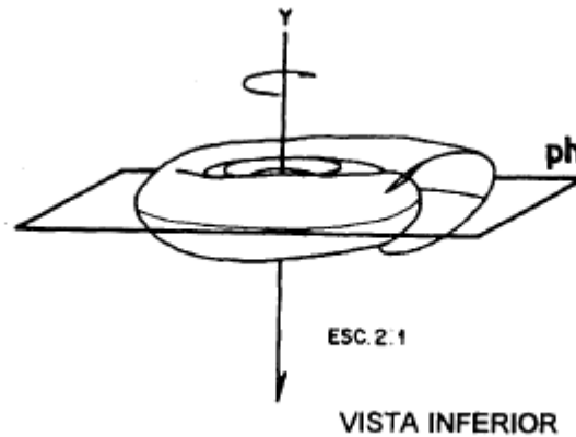
FIGURA 2: Morfologia externa da concha de Biomphalaria glabrata : ápice ( a ); umbigo ( u ); abertura da concha ( ac ); giro corporal ( gc ); peristoma ( p ); lábio direito ( ld ); lábio esquerdo ( le ); calo ( c ); suturas ( s )
