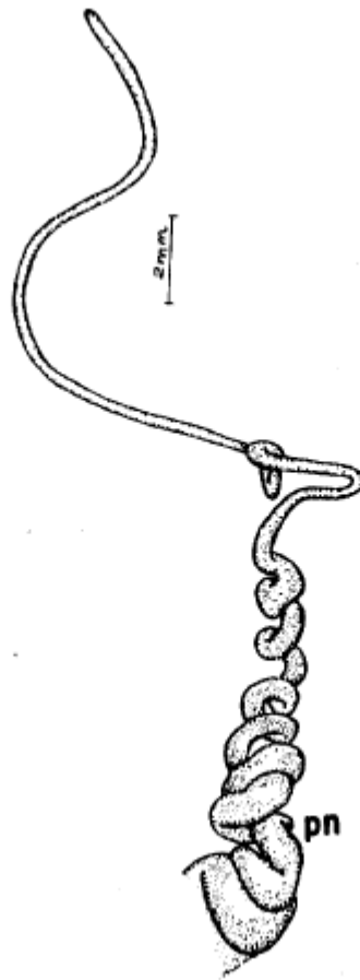
Figura 12. P. Lineata . Pênis parcialmente distendido: pn : pênis.
