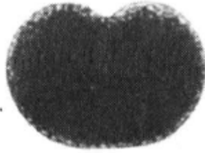
FIGURA 1-3: Sulco de clivagem, 4 minutos
