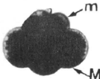
FIGURA 1-18/19: os blastômeros unidos, 173 e 181 minutos respectivamente
